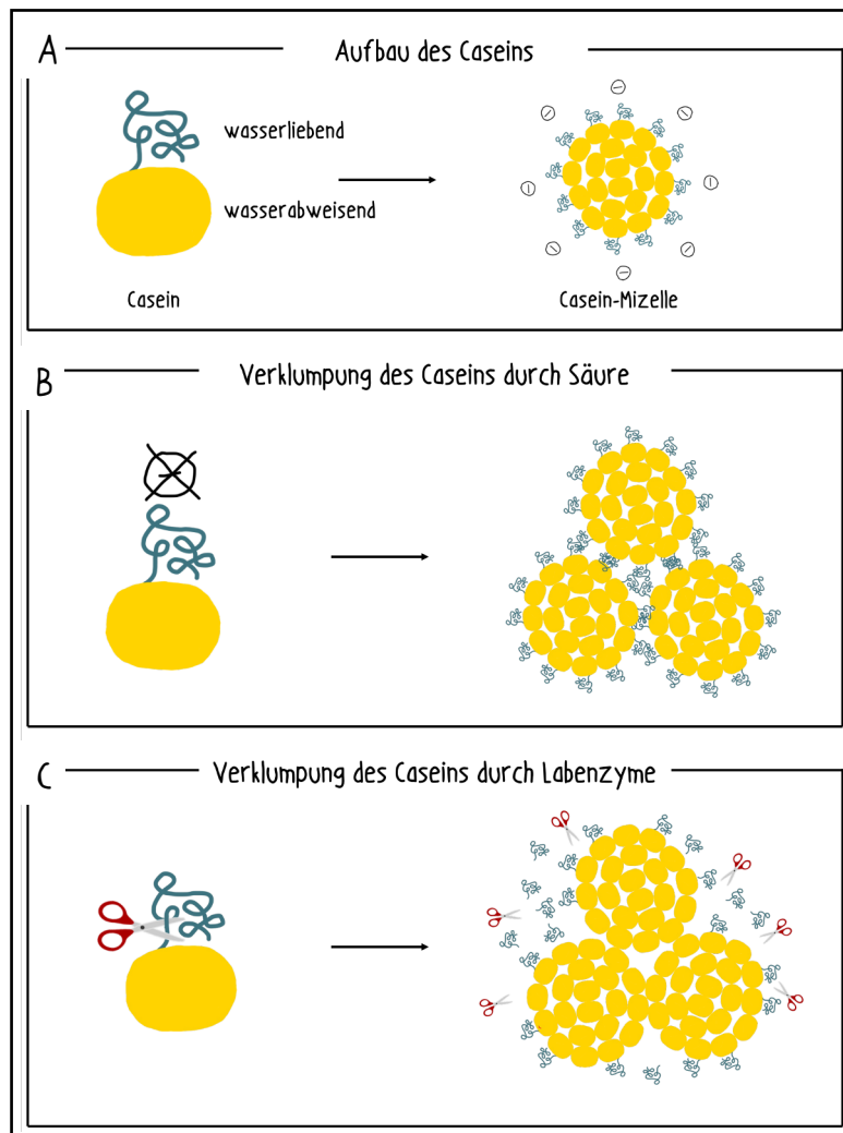
Bild 4: Casein verklumpt bei der Käseherstellung. A: Durch den wasserliebenden und wasserabweisenden Teil des Caseins lagert es sich zu Mizellen an. B: Durch Ansäuerung der Milch verliert Casein seine Ladung und die Mizellen lagern sich zusammen. C: Labenzyme schneiden den wasserliebenden Teil des Caseins ab, wodurch sich die Mizellen zusammenlagern.
